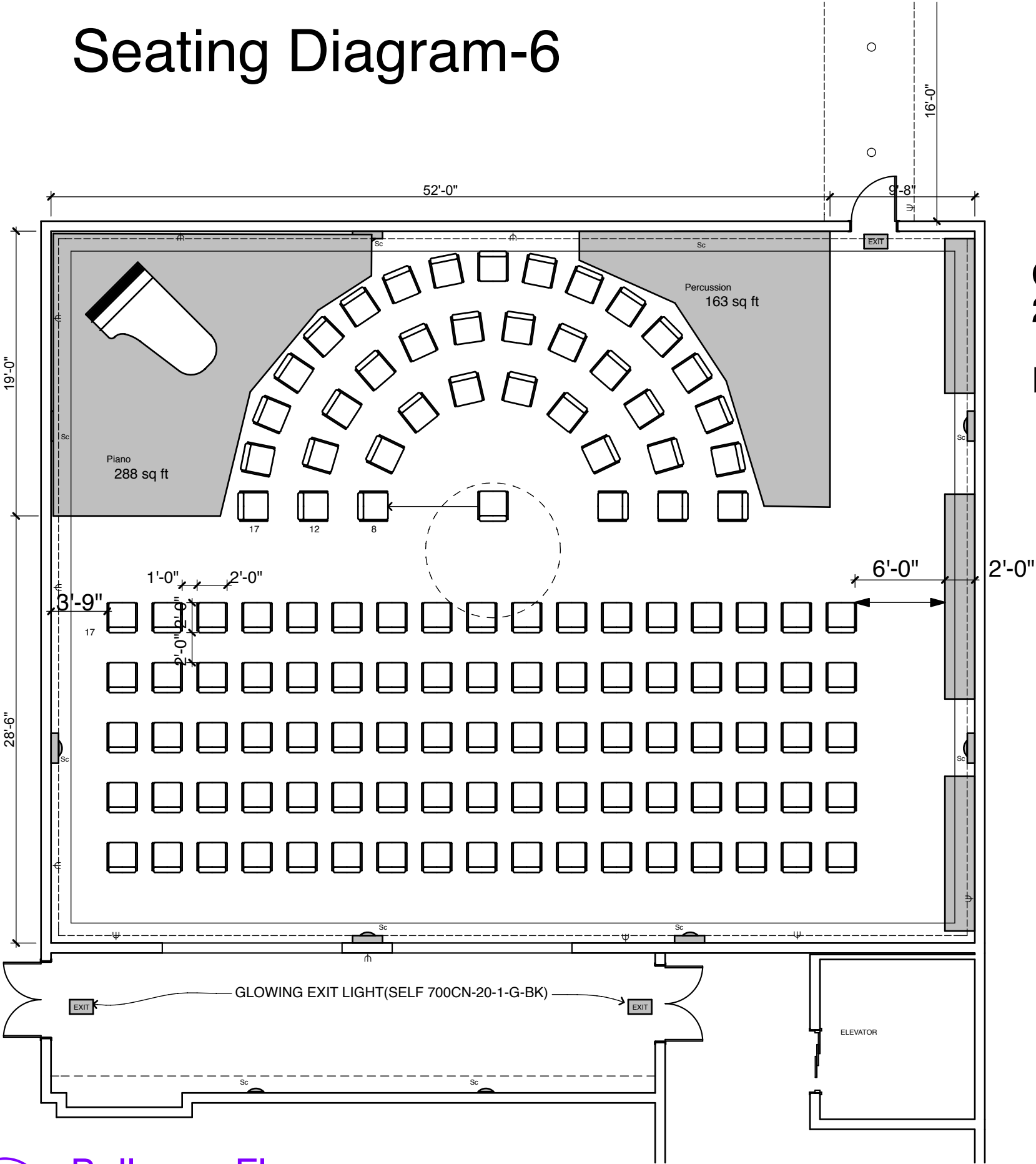
1 Ballroom Floor SCALE: 1/8" = 1'-0"
